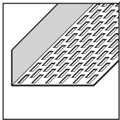
Profil perforé grille d'aération
